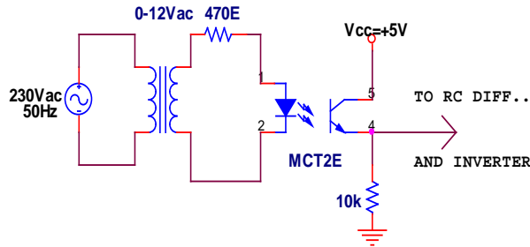
Fig.10: Opto-isolator (ZCD)
